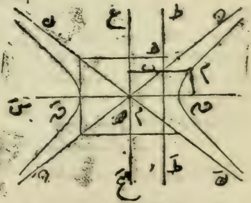
( قَطْع زَائِد ) \frac{m}{n} = 12.5
